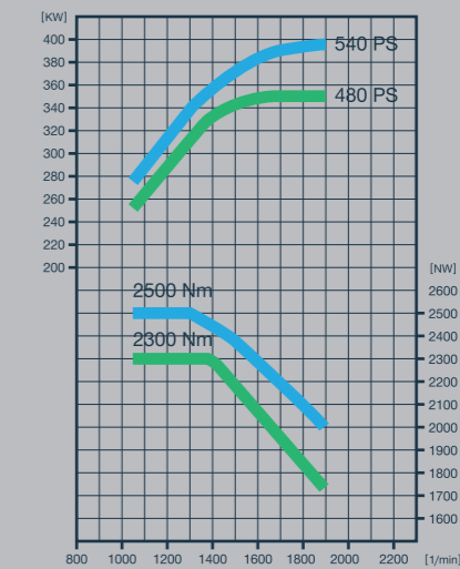
2.5 TGS engine data (2/2) D2066 / D2676
